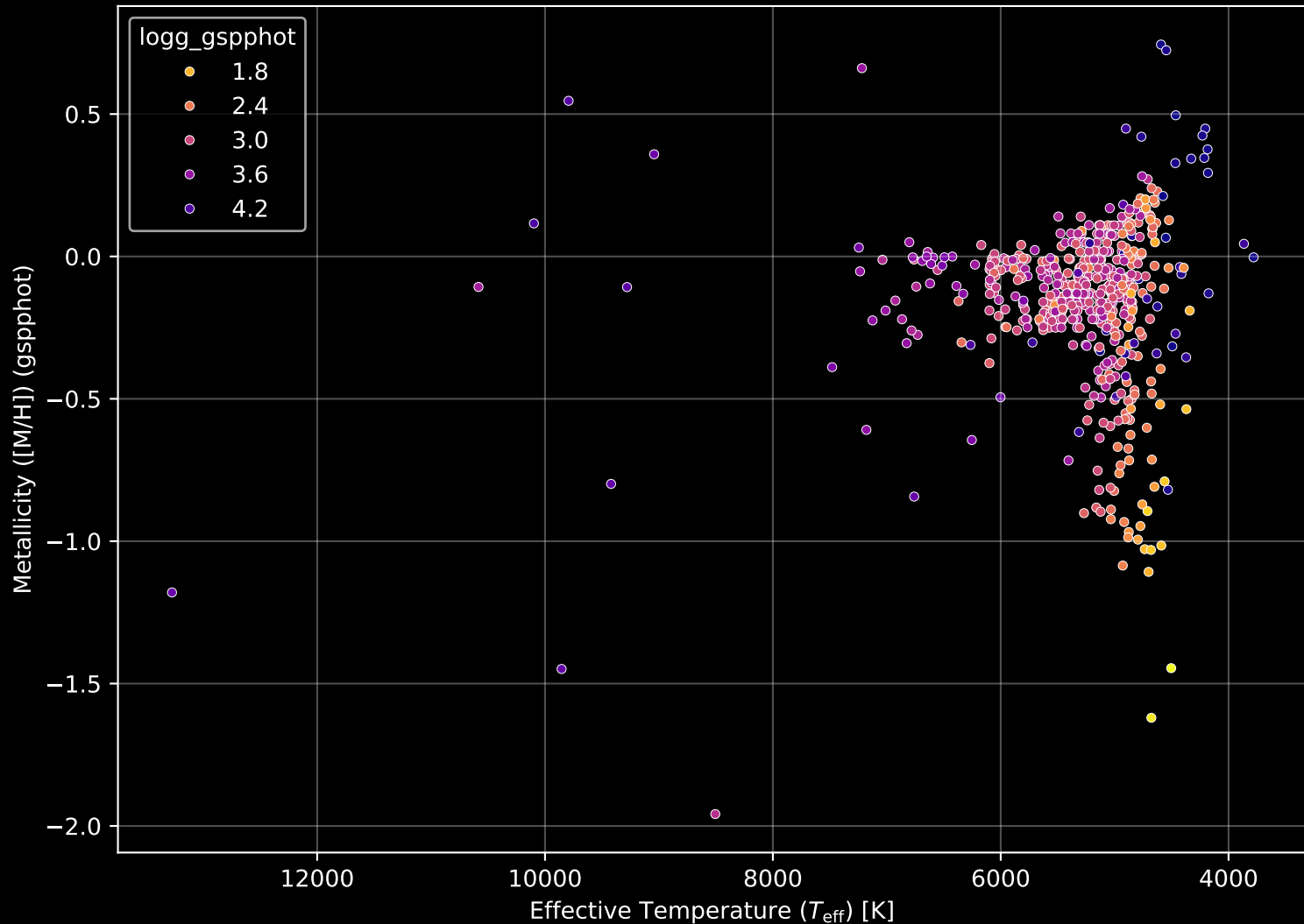
APOGEE DR17 Field: [251+00] Stellar Population Parameters (n= 559)
